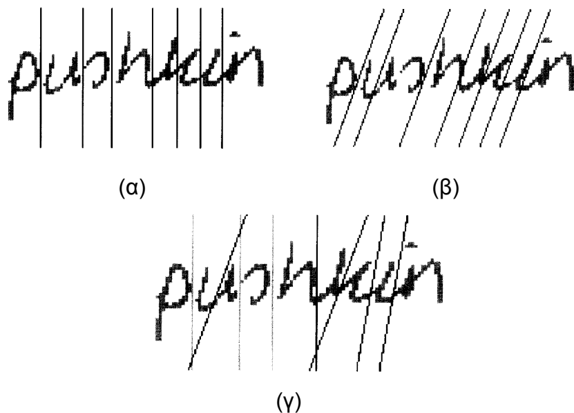
Σχήμα 2.41: (α)-(β) Κατάτμηση με διαχωριστικές γραμμές διαφορετικών κλίσεων, (γ) αποτέλεσμα που ενσωματώνει όλα τα αποτελέσματα κατάτμησης μαζί με το τελικό αποτελέσματα.
