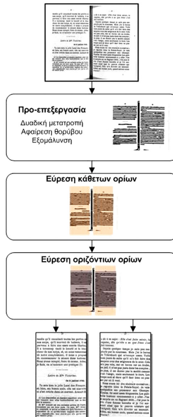
Σχήμα 3.7: Διάγραμμα ροής προτεινόμενης μεθόδου για τον εντοπισμό και την αφαίρεση του περιθωρίου καθώς και τον διαχωρισμό των διπλών σελίδων.
