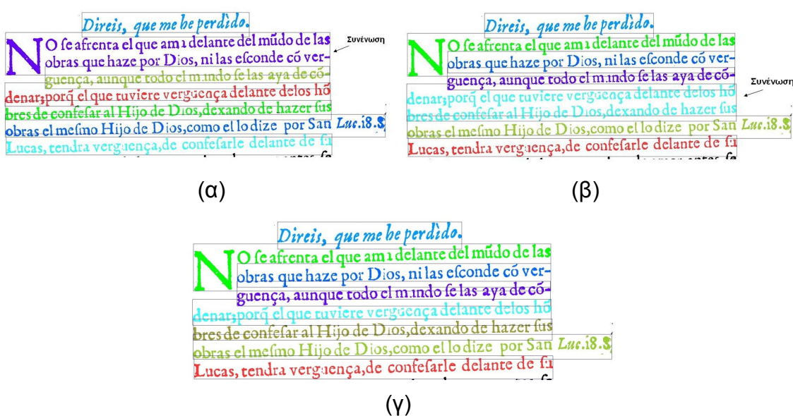
Σχήμα 5.12: Αποτελέσματα κατάτμησης ιστορικής εικόνας εγγράφου με τη χρήση της μεθόδου (α) ανάλυσης προβολών [77], (β) adaptive RLSA [115] και (γ) μετά τον συνδυασμό τους.
